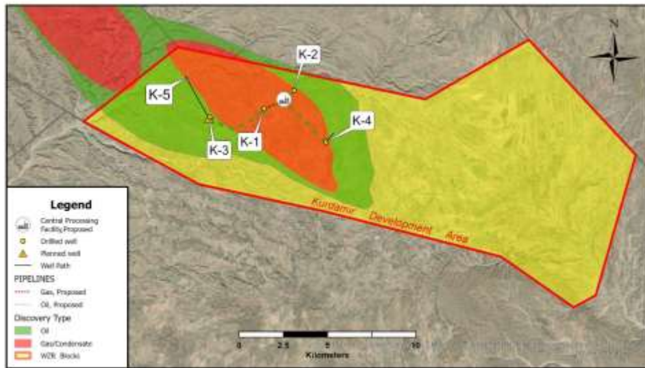
ناوچە ی پەرەپێدانی کوردە میر
